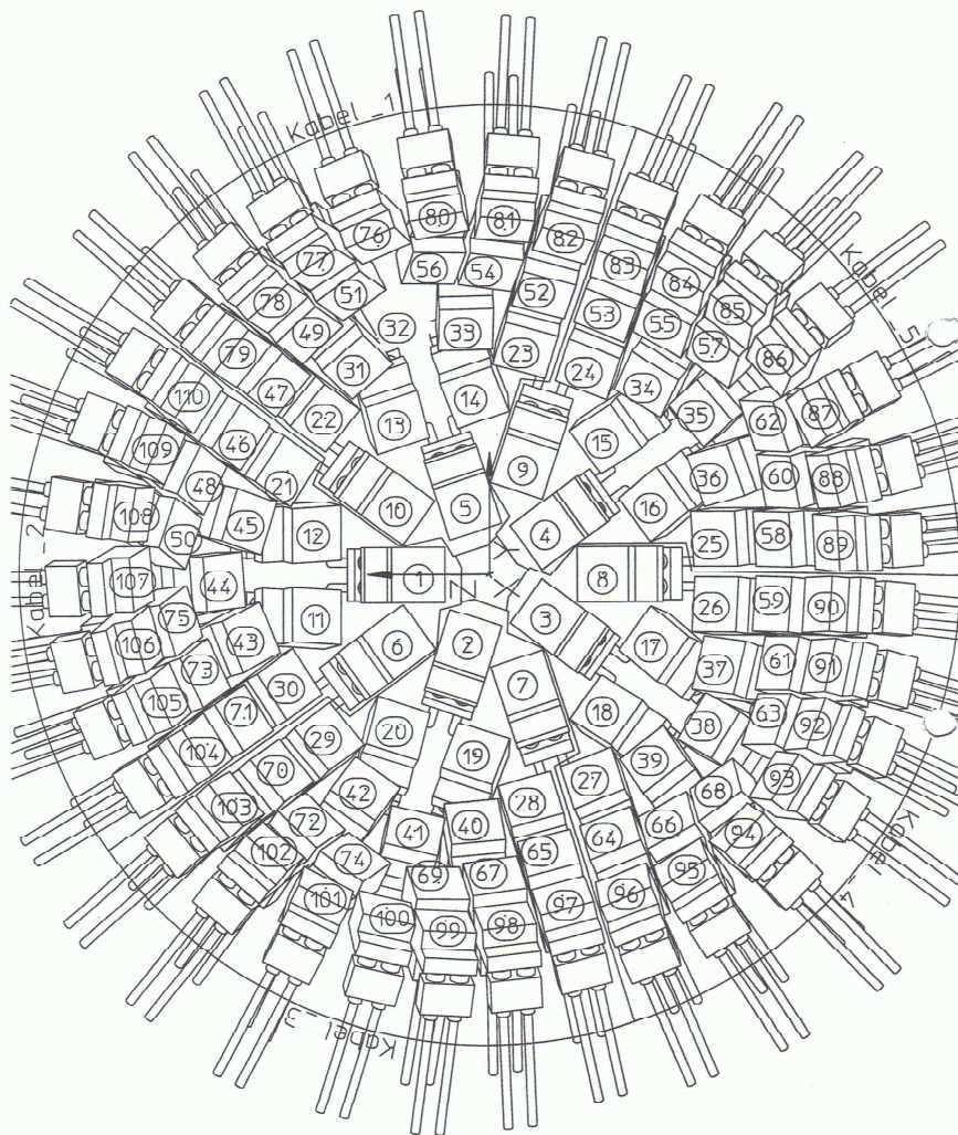
296.02.003.4 Zusammenfassung der Verkabelungsgruppen Nordball_2D_296.02.002-4.4
